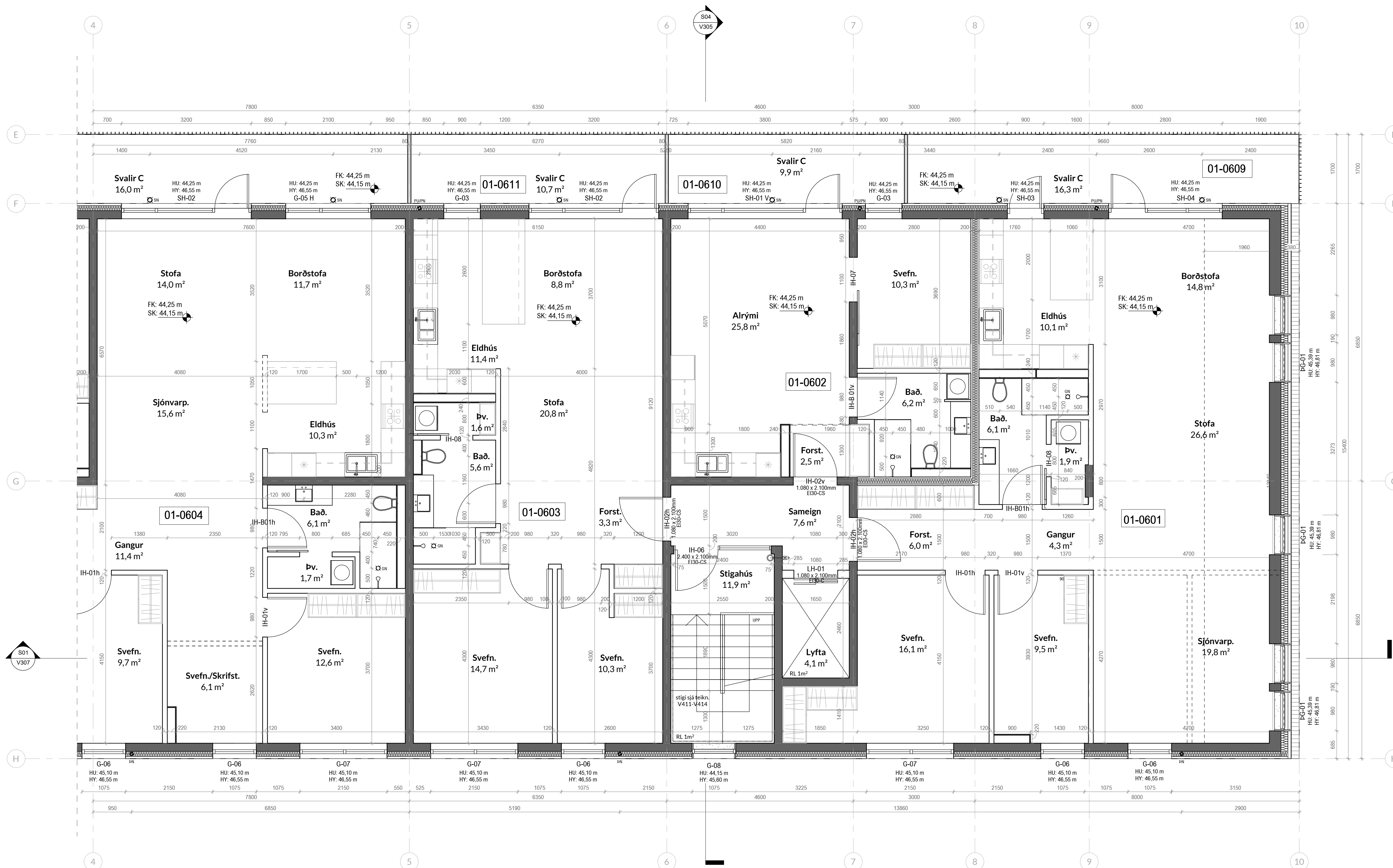
Mhl.01 6.hæð. - b 1:50
