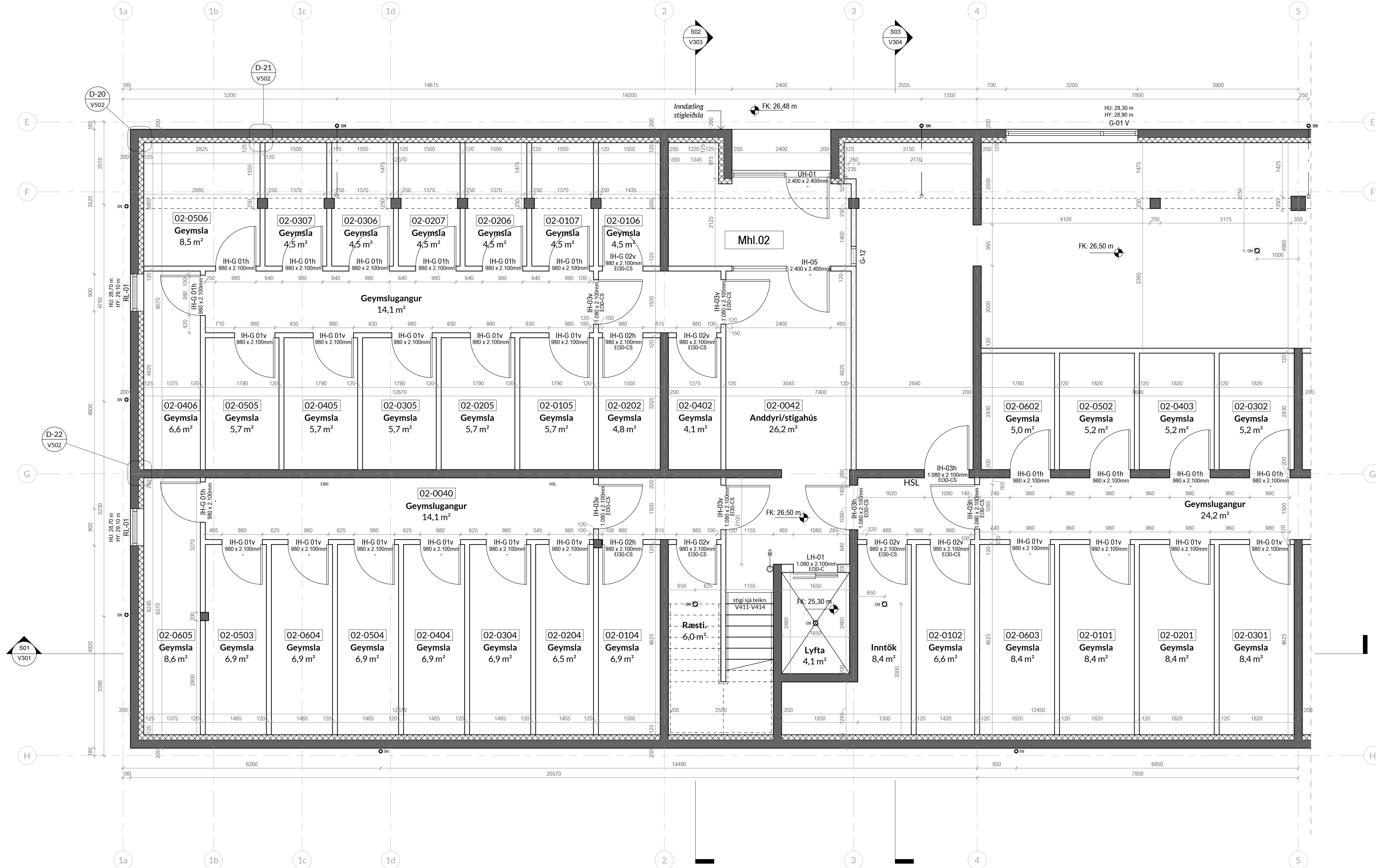
Mhl.02 Kjallari - a 1:50
