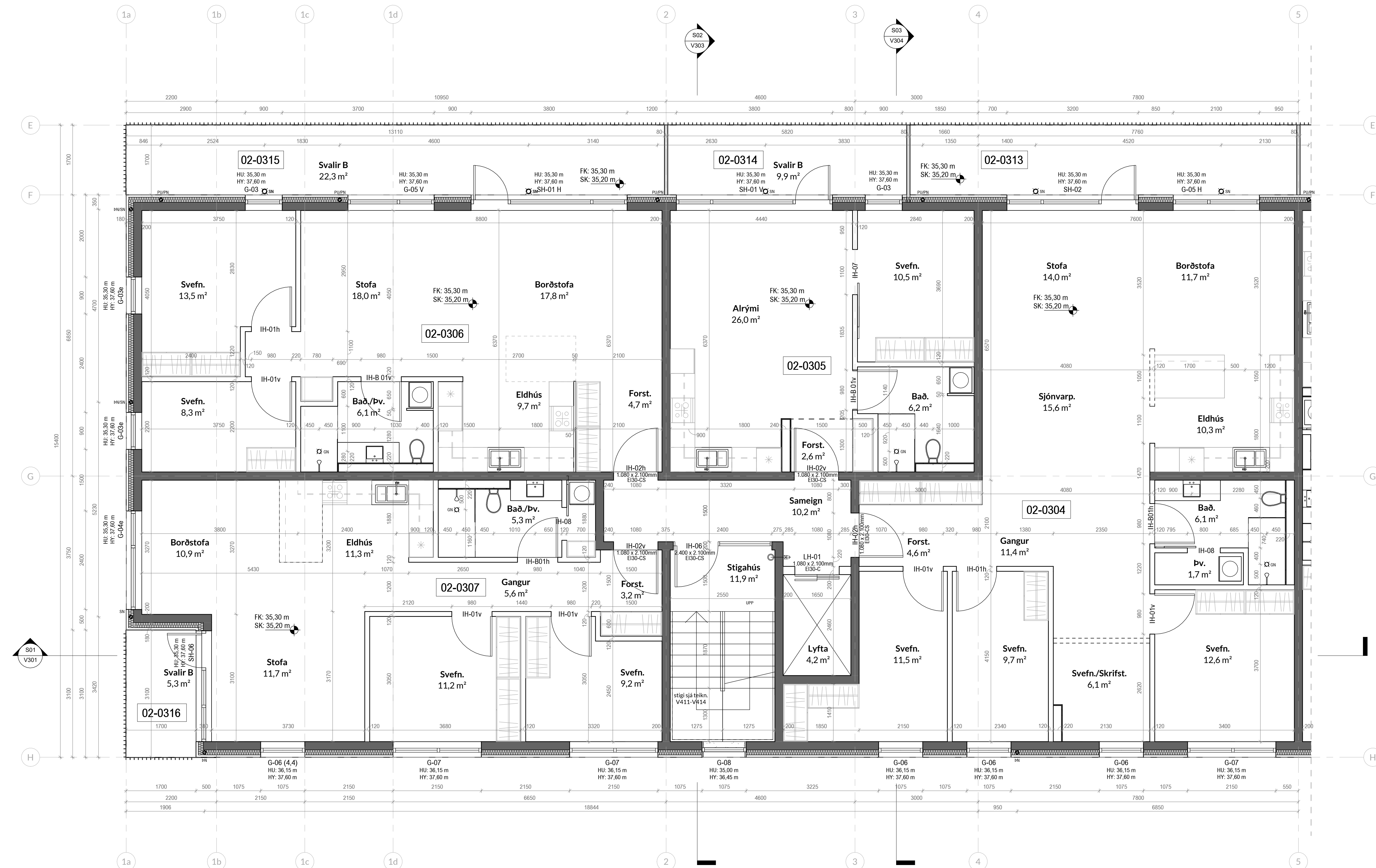
Mhl.02 3.hæð - a 1:50
