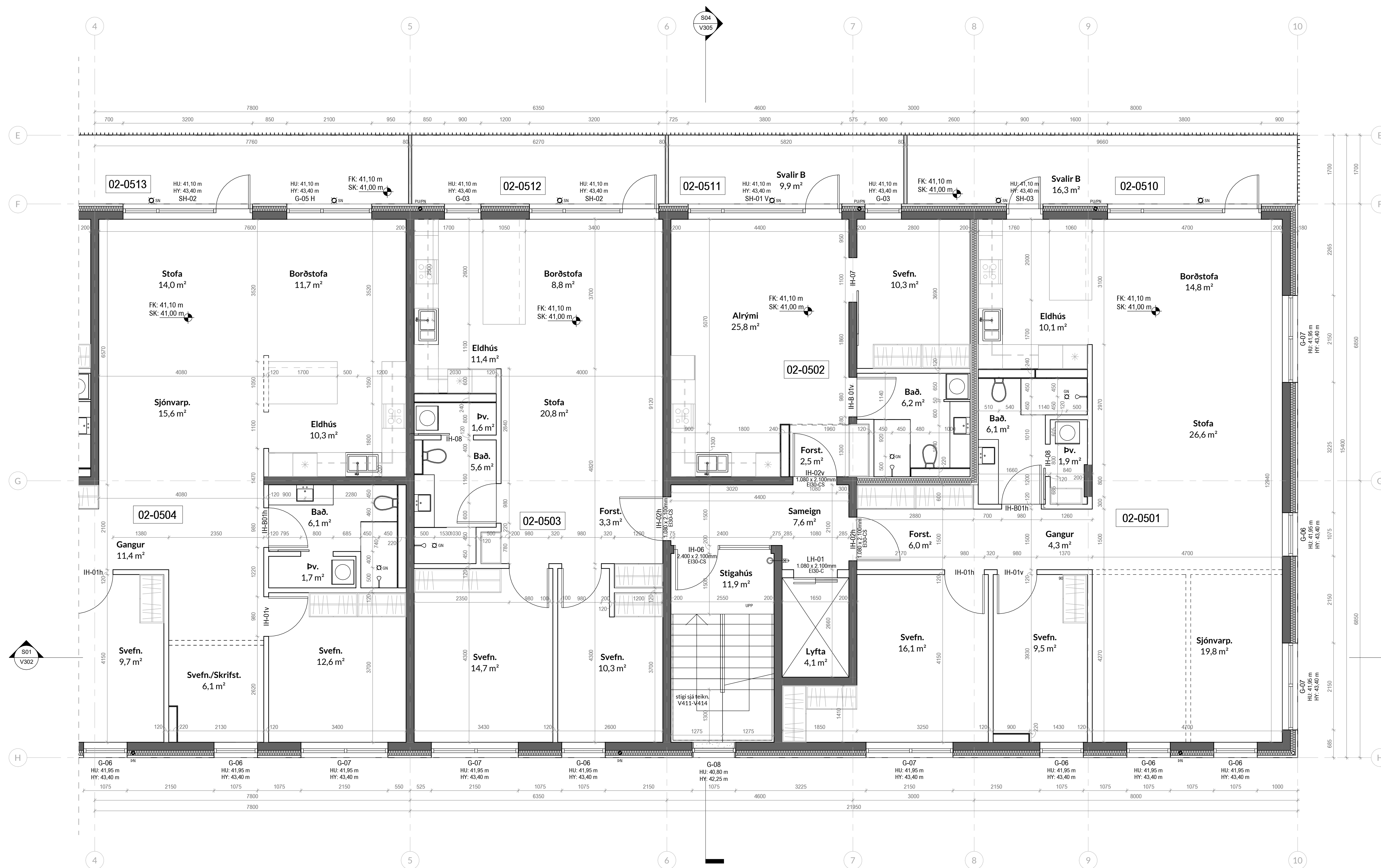
Mhl.02 5.hæð. - b 1:50
