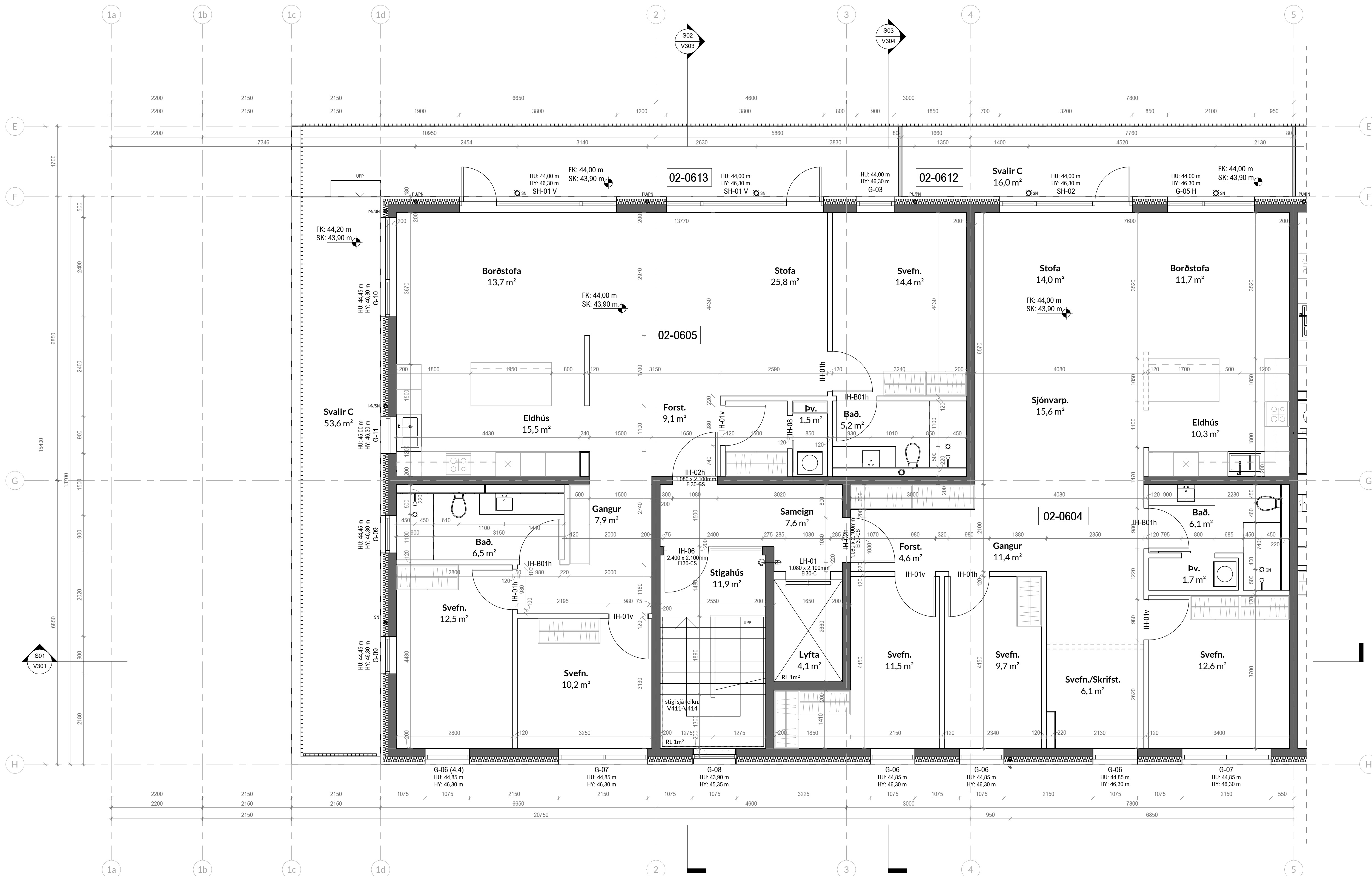
Mhl.02 6.hæð. - a 1:50
