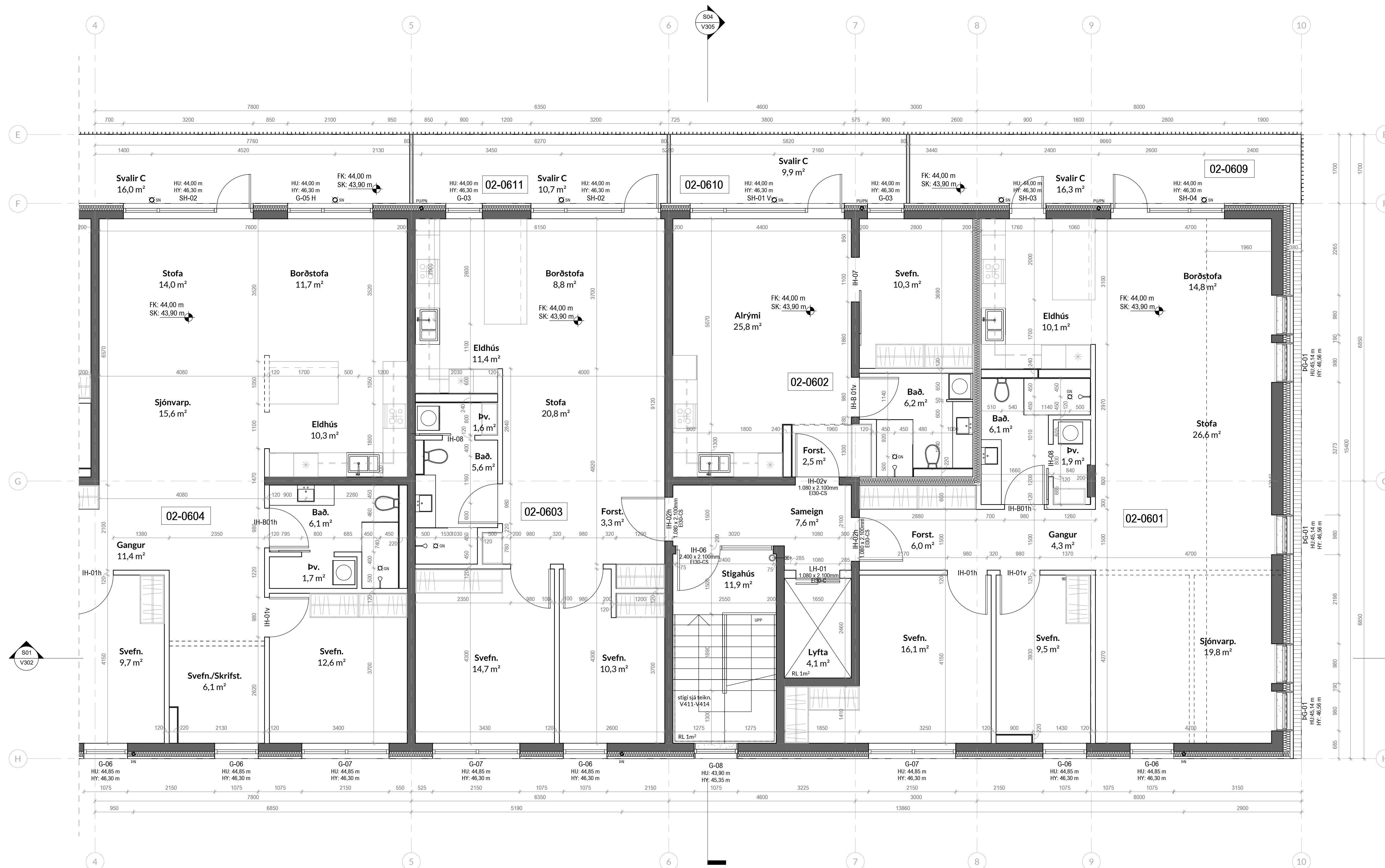
Mhl.02 6.hæð - b 1:50
