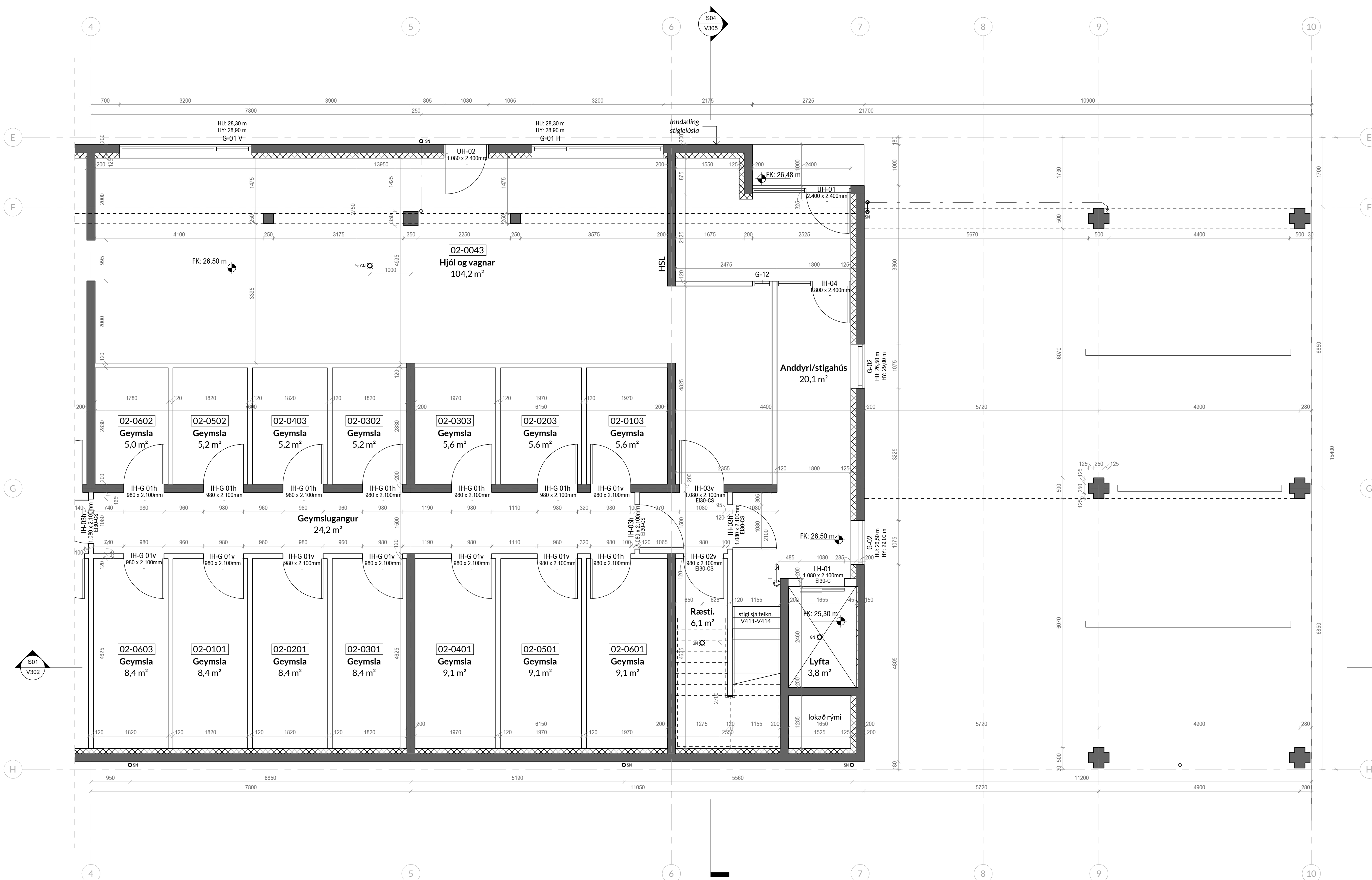
Mhl.02 Kjallari. - b 1:50
