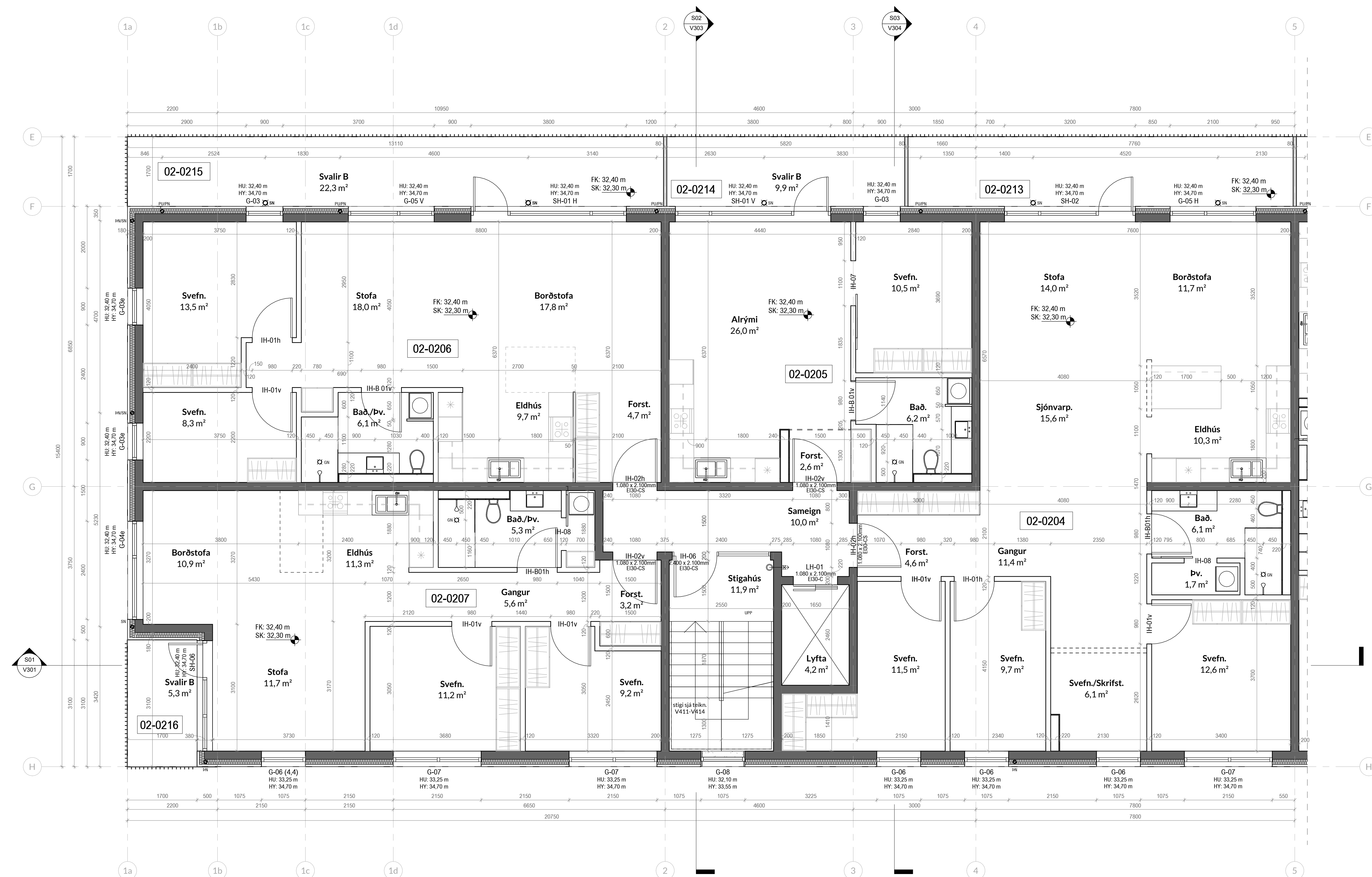
Mhl.02 2.hæð. - a 1:50
