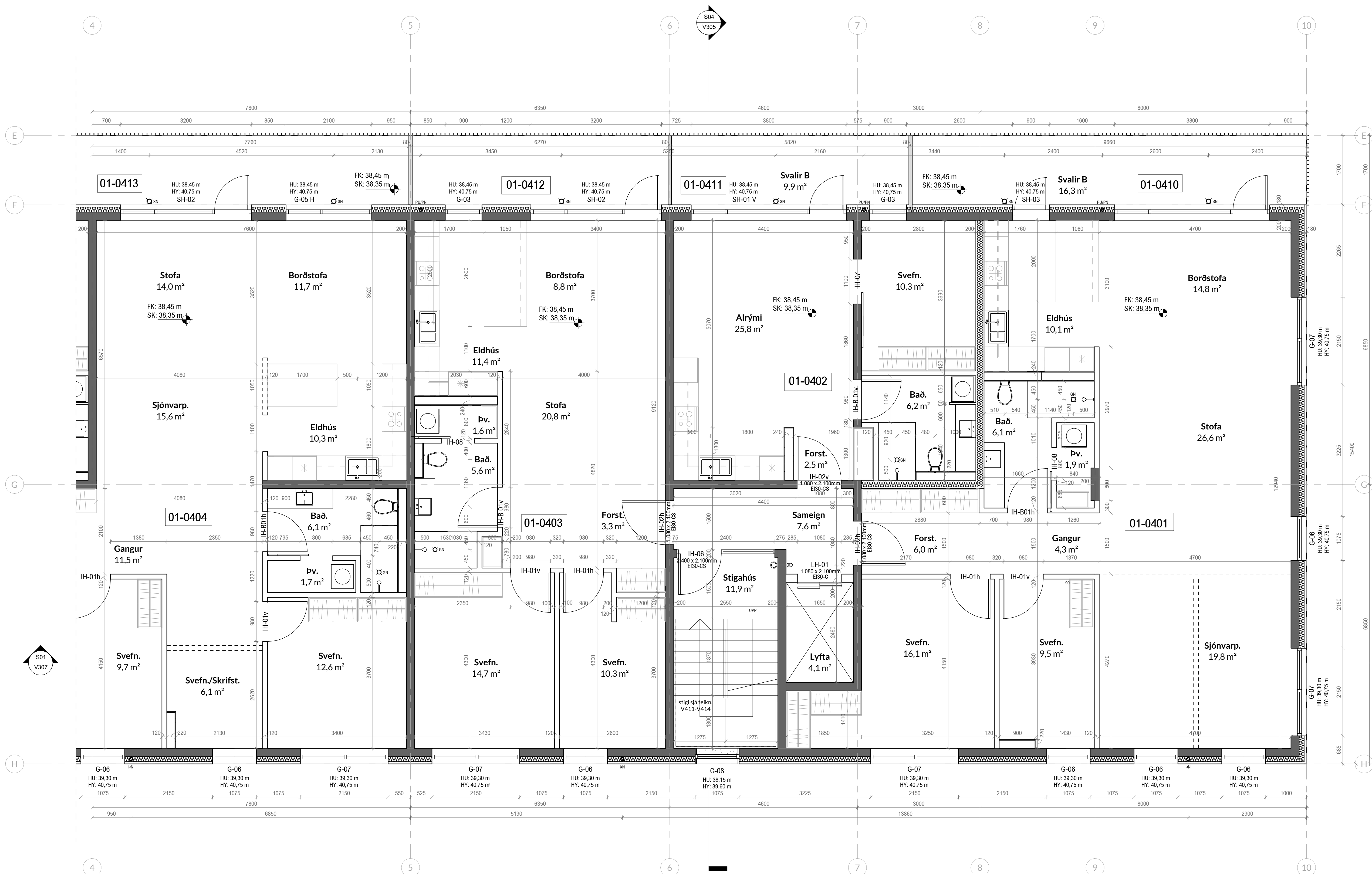
Mhl.01 4.hæð. - b 1:50
