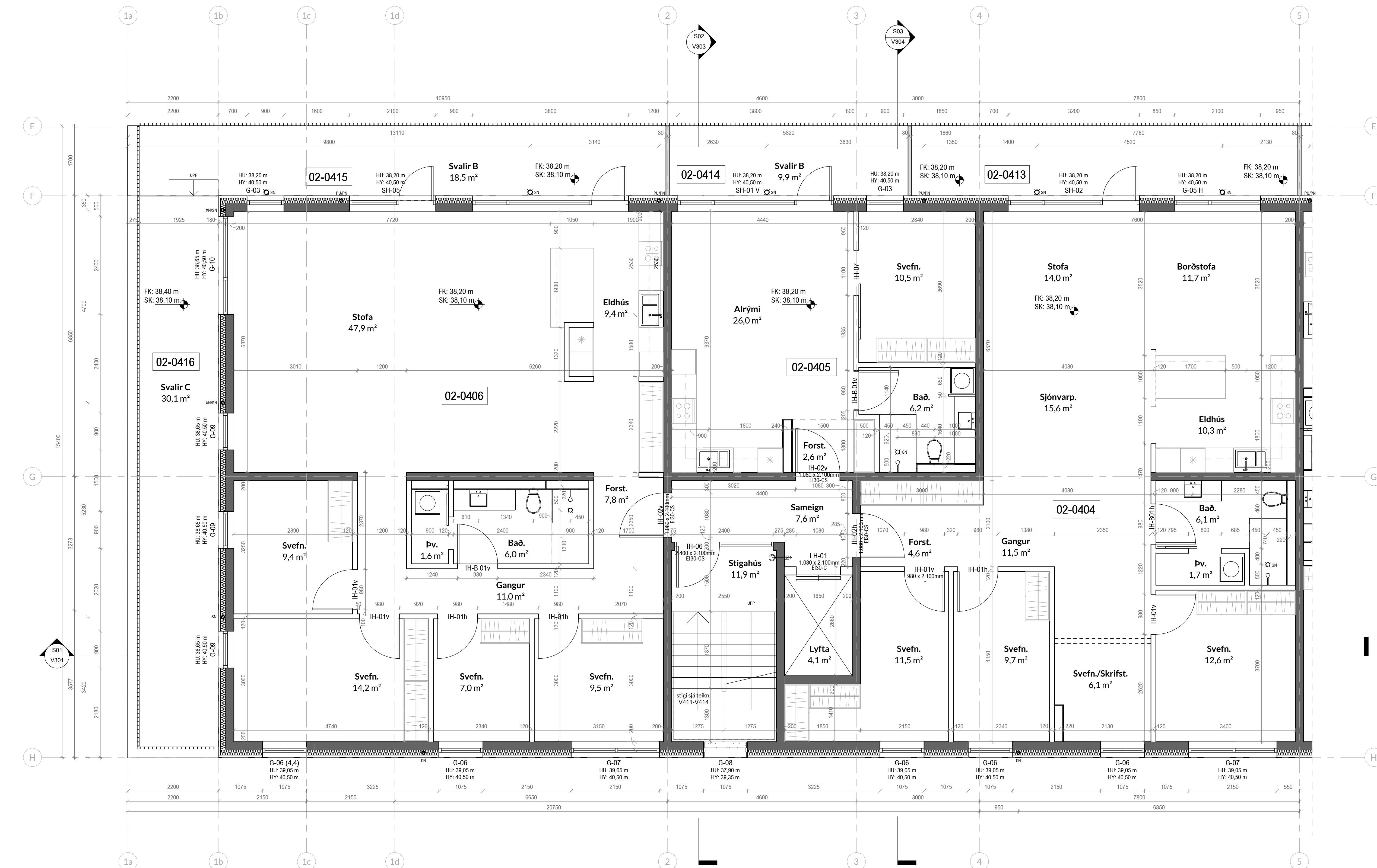
Mhl.02 4.hæð - a 1:50
