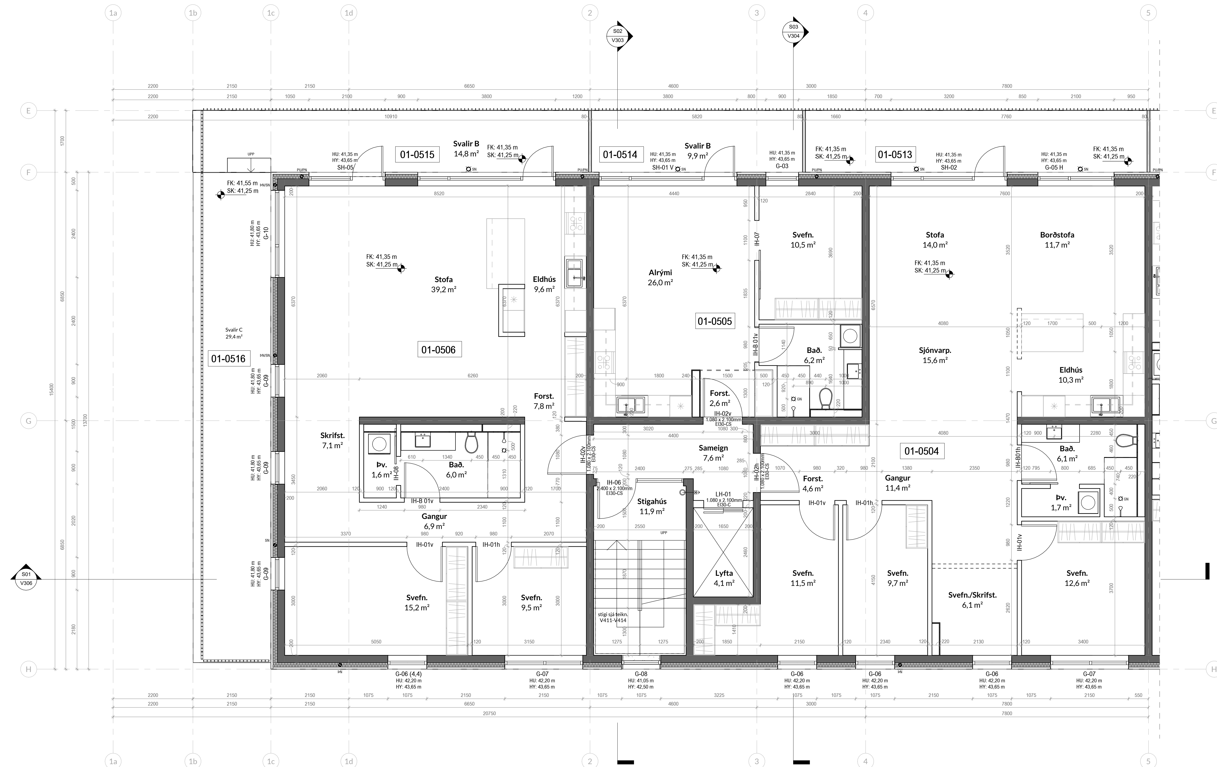
Mhl.01 5.hæð. - a 1:50
