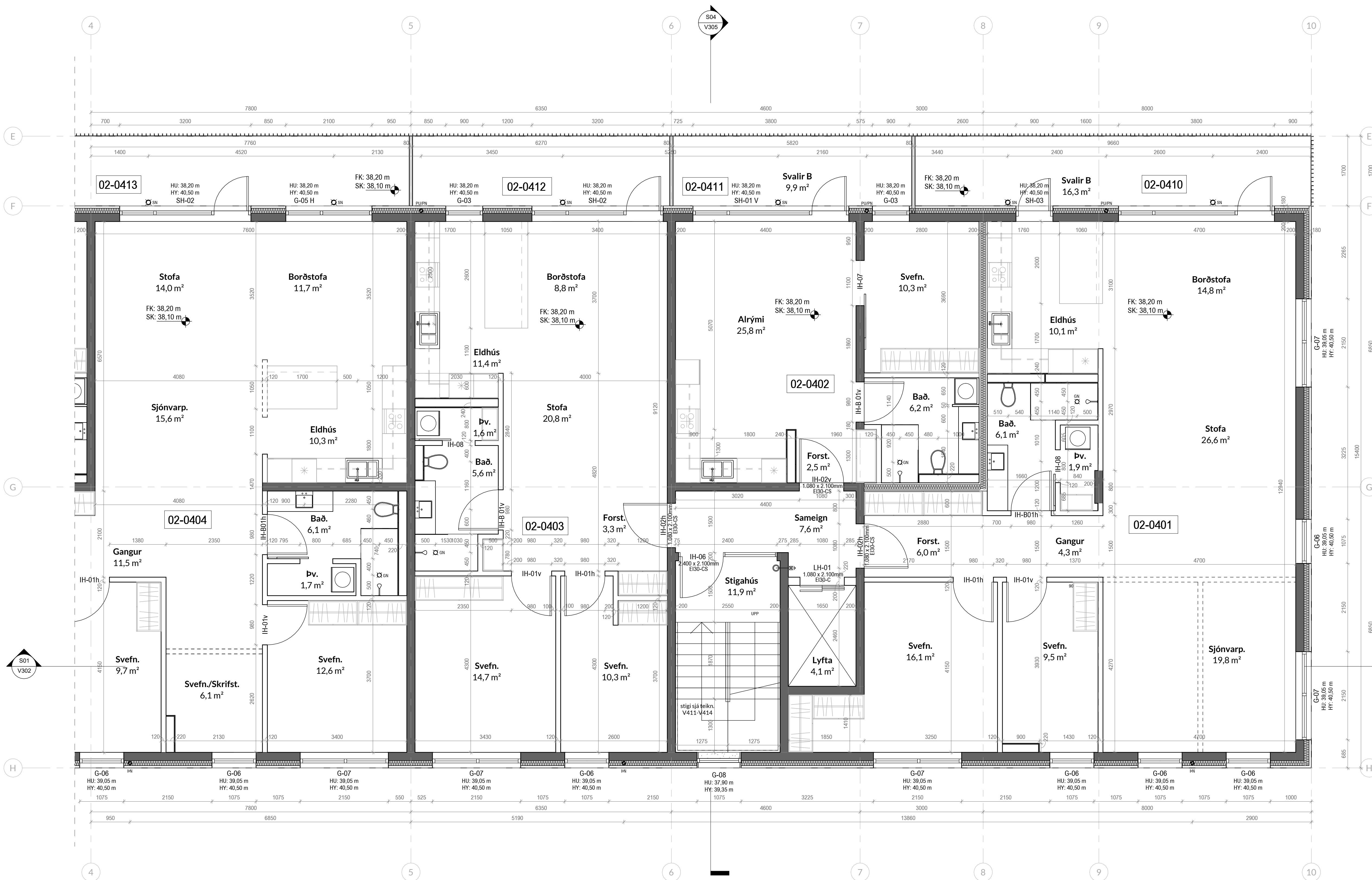
Mhl.02 4.hæð - b 1:50
