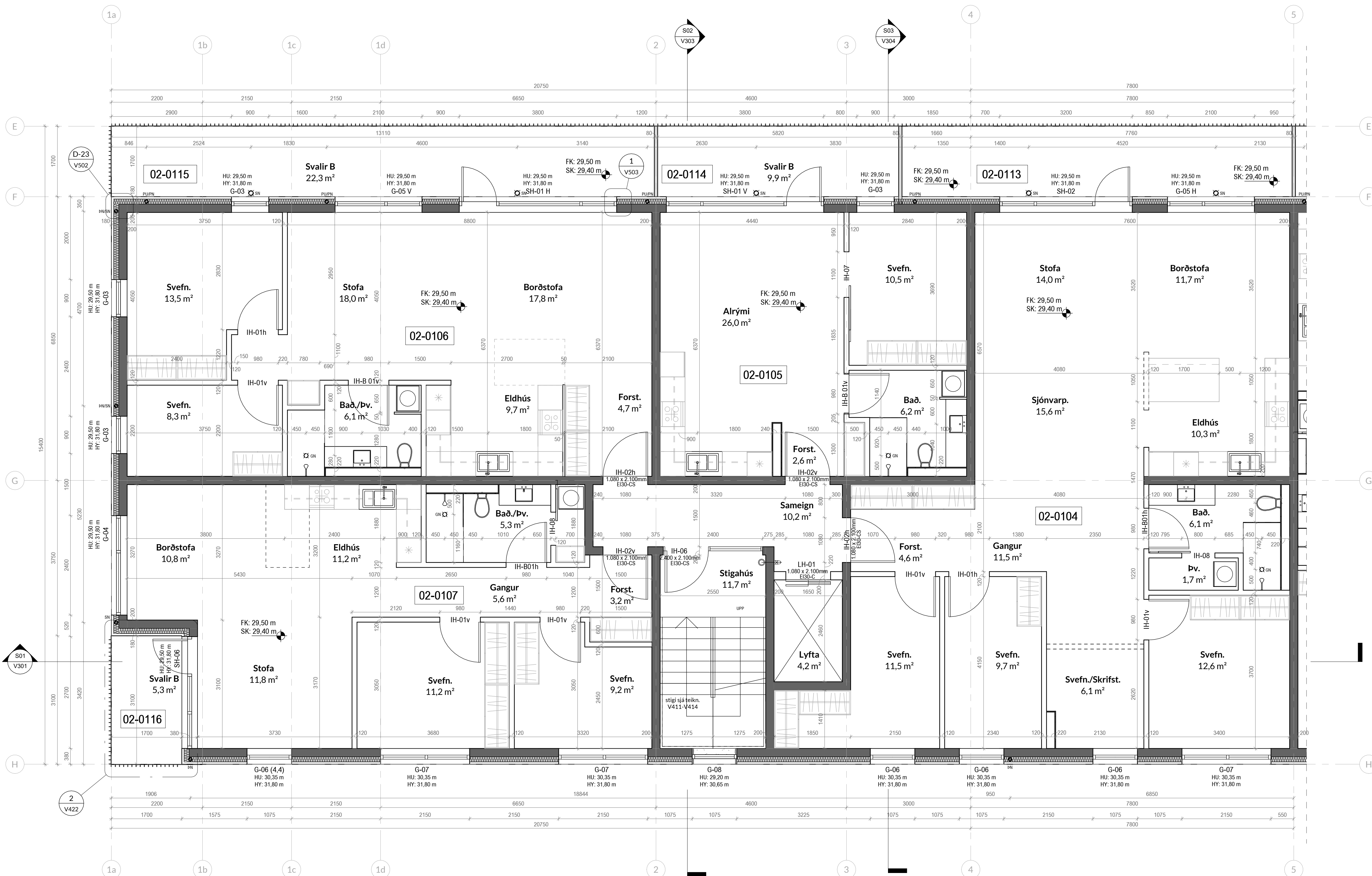
Mhl.02 1.hæð. - a 1:50
