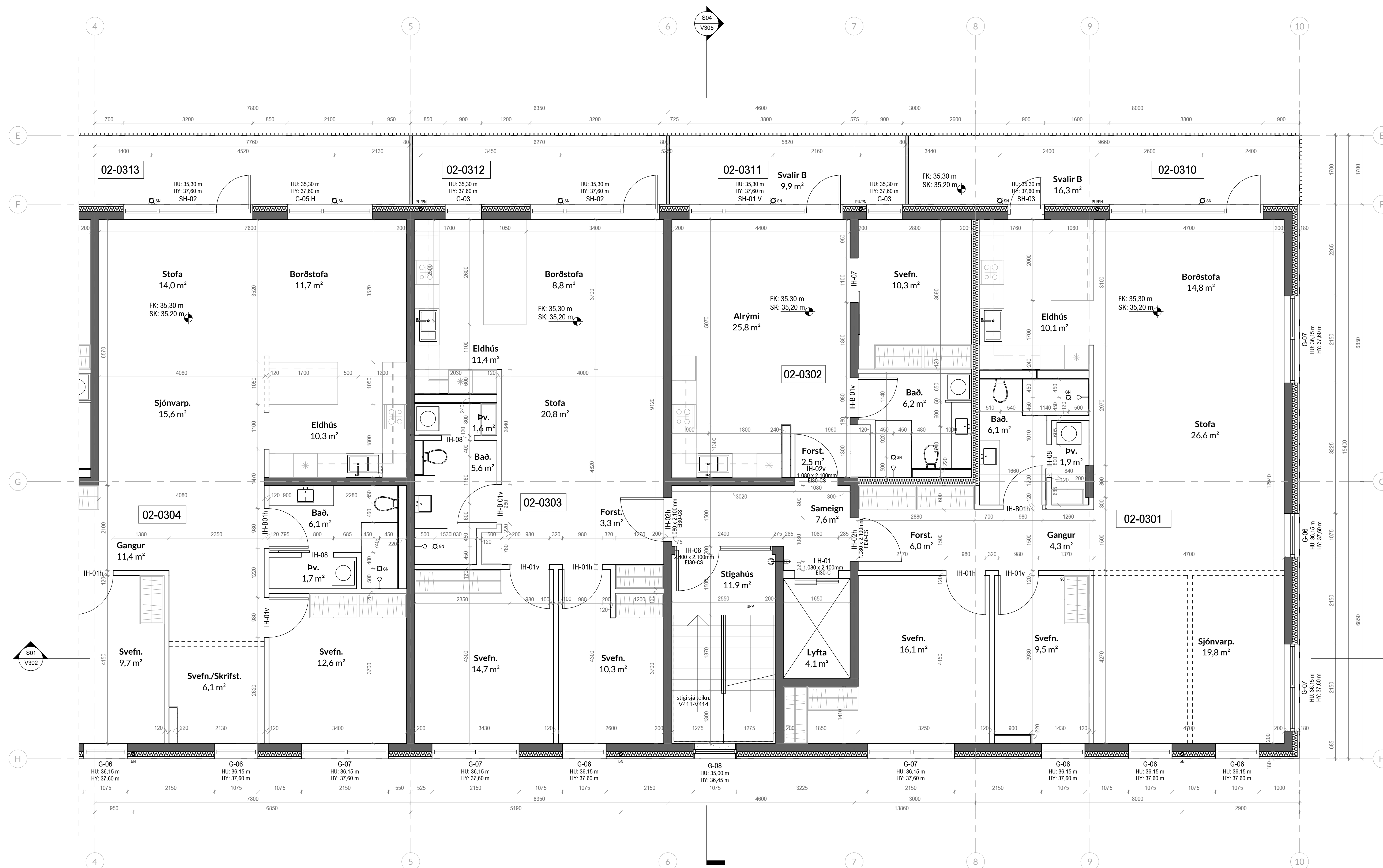
Mhl.02 3.hæð. - b 1:50
