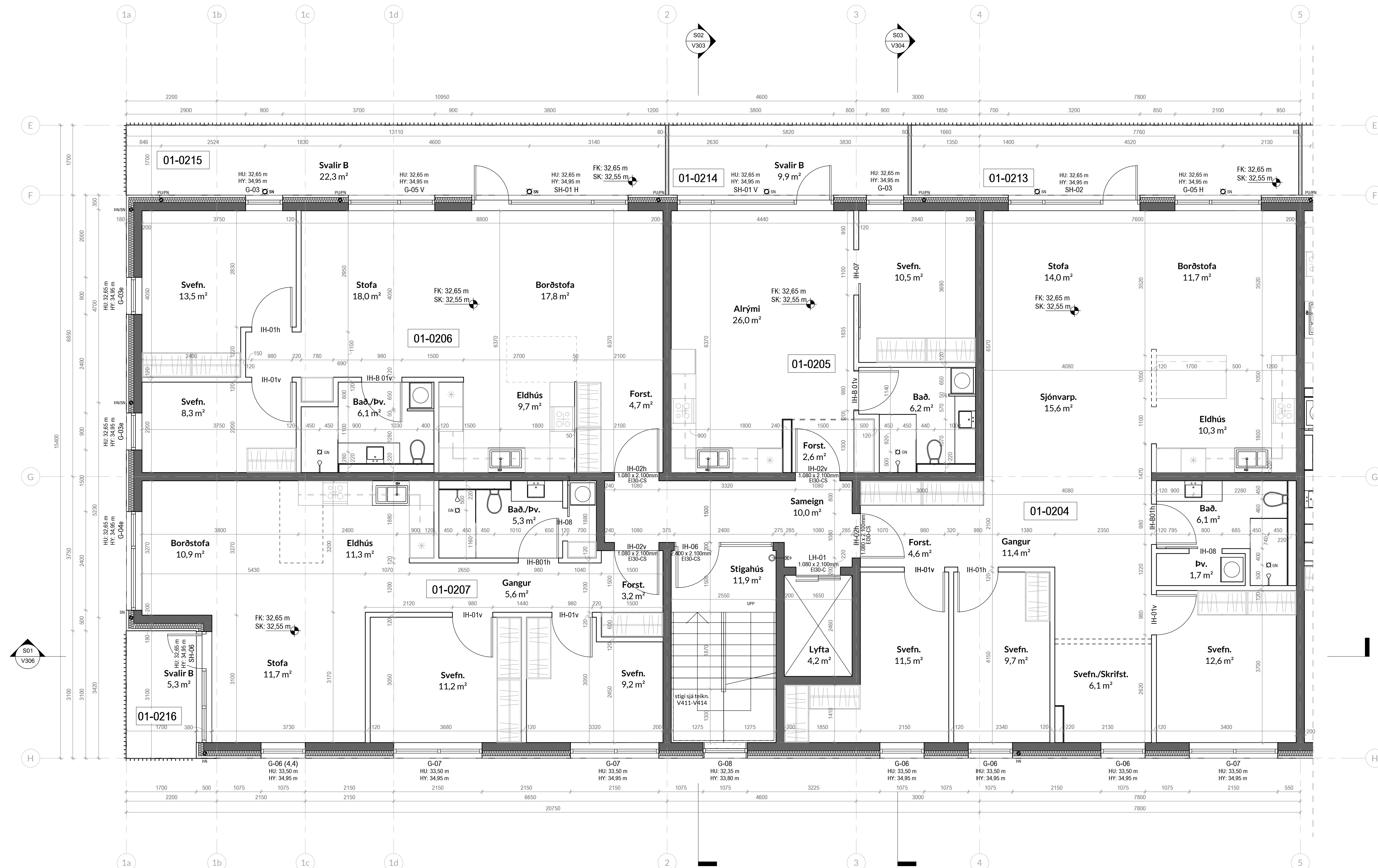
Mhl.01 2.hæð. - a 1:50
