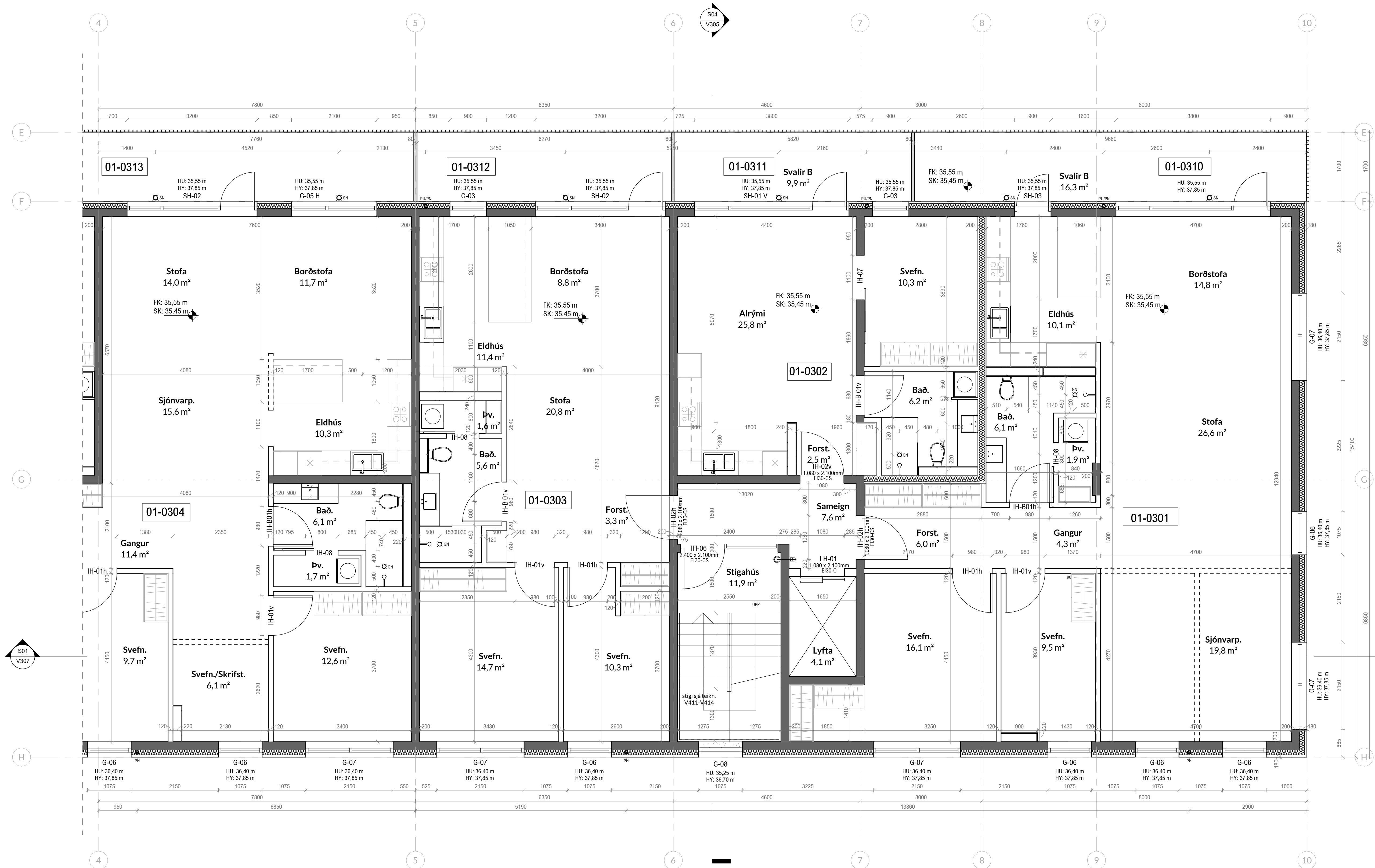
Mhl.01.3.hæð. - b 1:50
