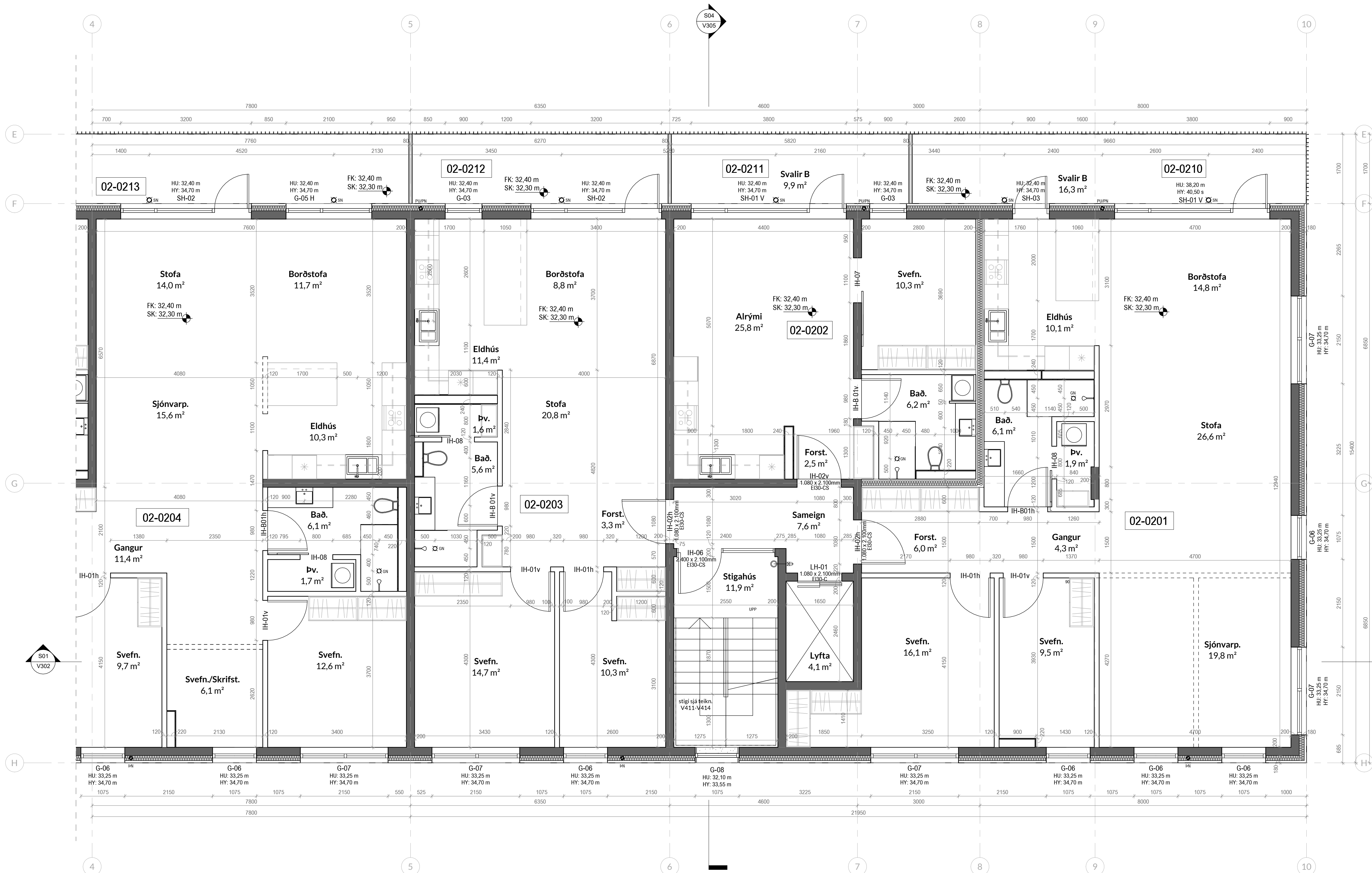
Mhl.02.2.hæð. - b 1:50
