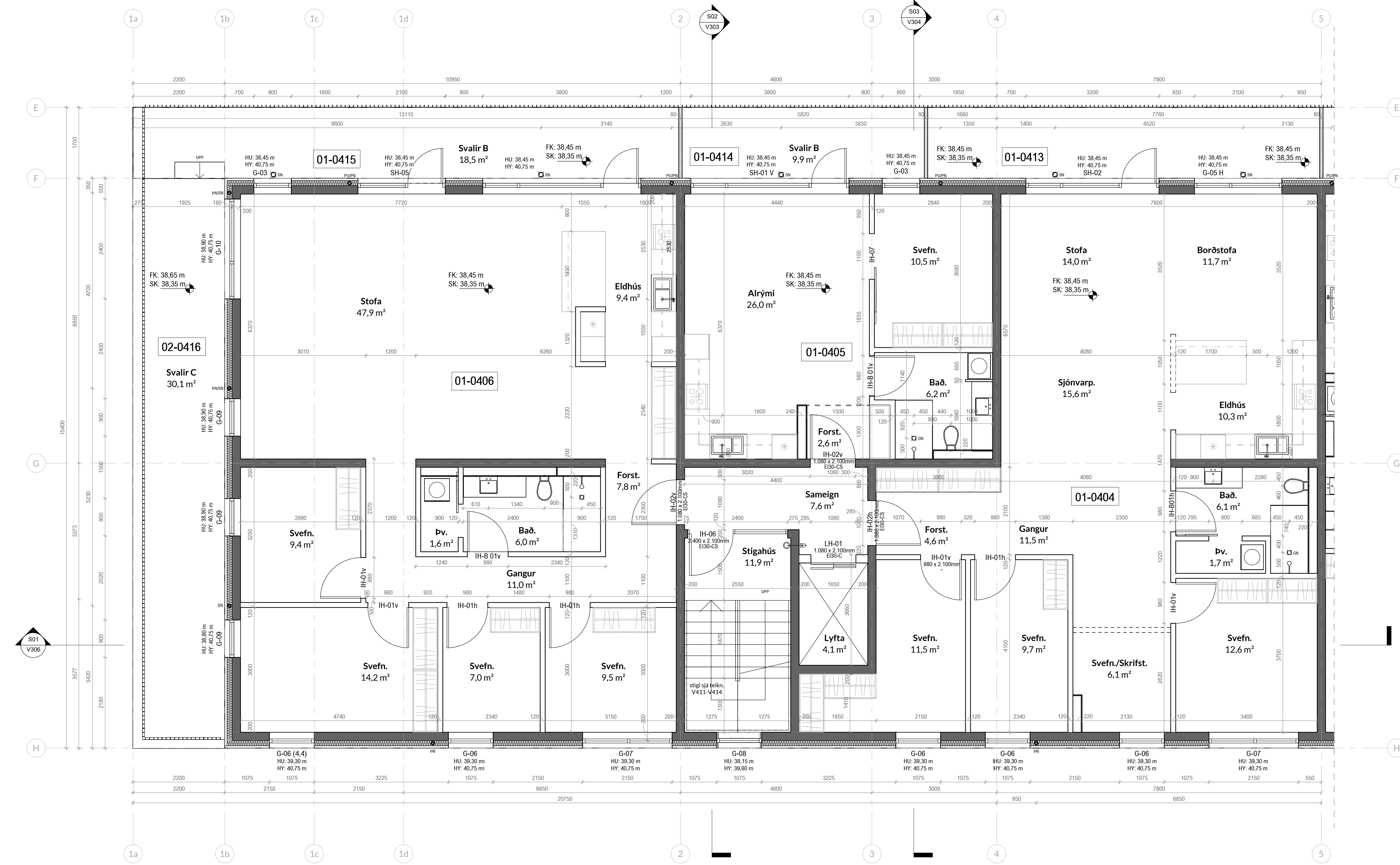
Mhl.01 4.hæð. - a 1:50
